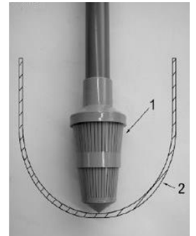
Bild 1: Steigrohr mittig
